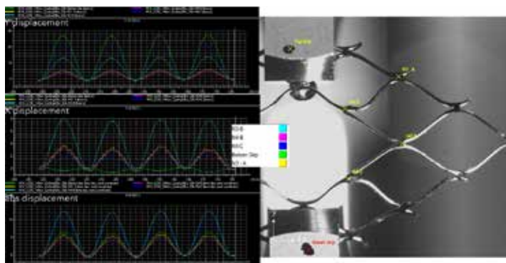
Skärmbild av TEMA Pro när den används av Medtronic för att utvärdera rörelsemönster hos en aortastentgraft.
